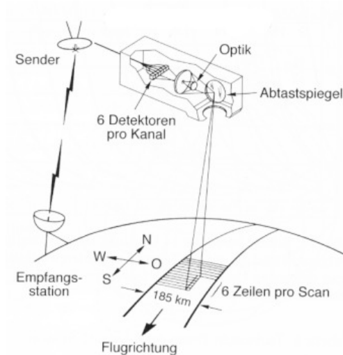
Schematische Darstellung der Aufnahme mit dem Landsat MSS-System [Albertz 2001]
