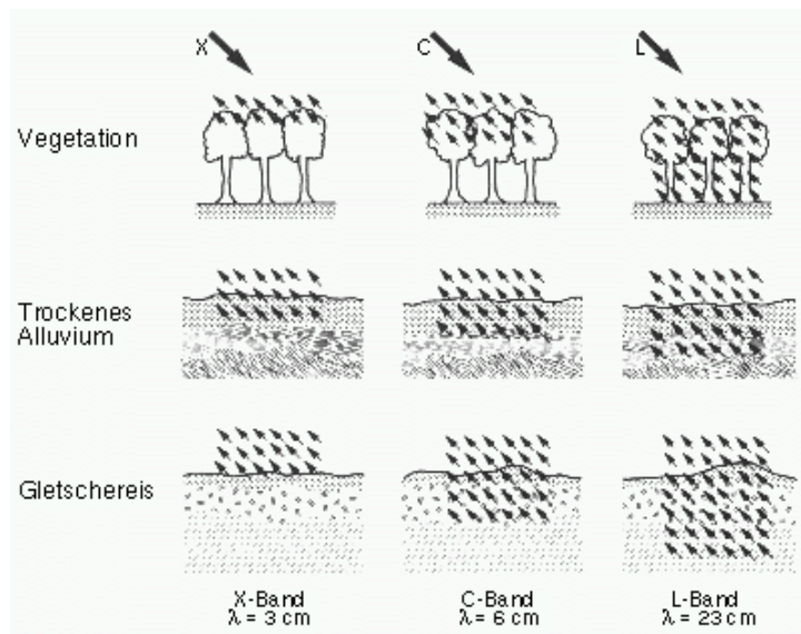
Wechselwirkung zwischen Mikrowellen und Erdoberfläche in Abhängigkeit von Wellenlänge und Leitfähigkeit [Albertz 2001]
