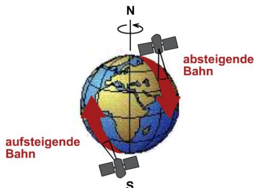
Aufsteigende und absteigende Bahn eines polarumlaufenden Satelliten
