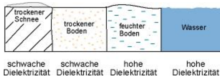
Dielektrizität verschiedener Objekte der Erdoberfläche
