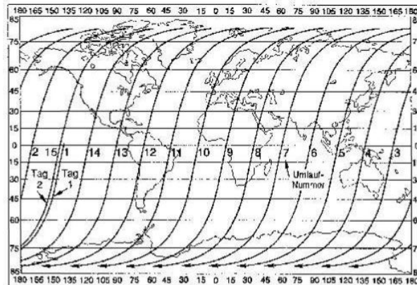
Bodenspuren für die Satelliten Landsat 1-3 [Albertz 2001]
