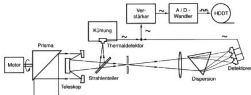
Funktionsweise eines opto-mechanischen Scanners [Albertz 2001]
