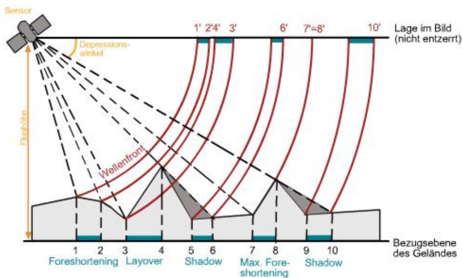
Fehler in Radarbildern: Foreshortening, Layover und Radarschatten
