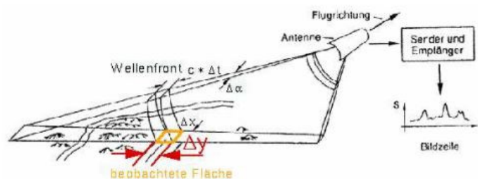
Schematische Darstellung eines SLAR [Albertz 2001]
