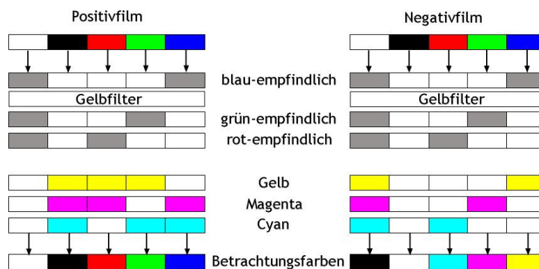
Positiv- und Negativfilm
