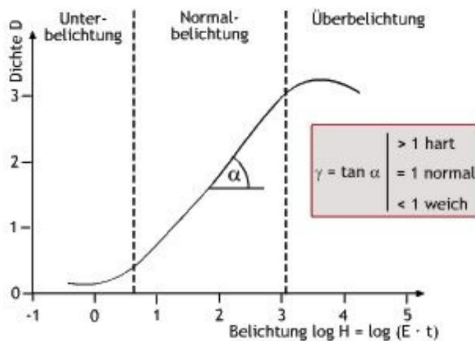
Schwärzungskurve: Zusammenhang zwischen Dichte und Belichtung
